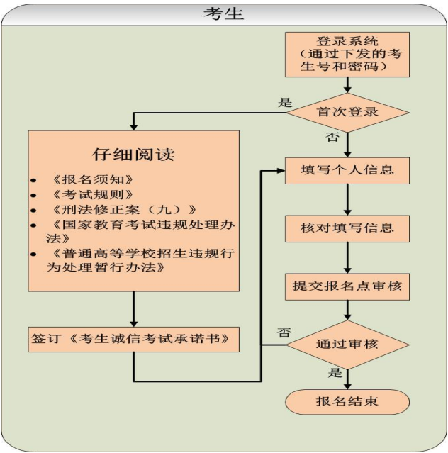
图 1.1 业务流程图
